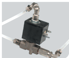
Electroválvula de mezcla para garantizar temperaturas diferenciadas e ideales de los productos solubles.
